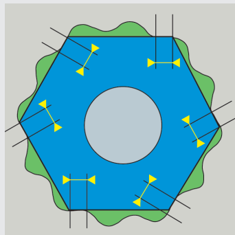
POWERDRIV® használatával: felületen átadódó nyomás
