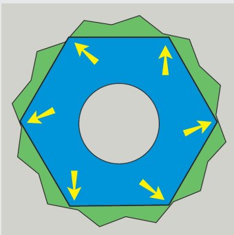
POWERDRIV® nélkül: vonalban átadódó nyomás
